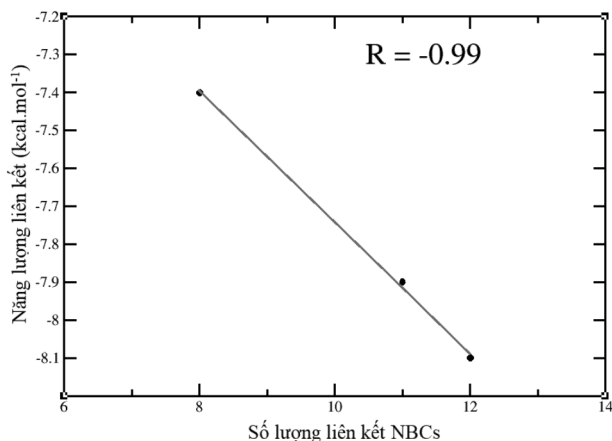
Hình 6. Tương quan giữa năng lượng liên kết và số lượng liên kết NBCs
